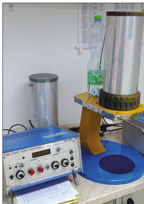
Spektrometr pro měření velkých scintilačních komor
